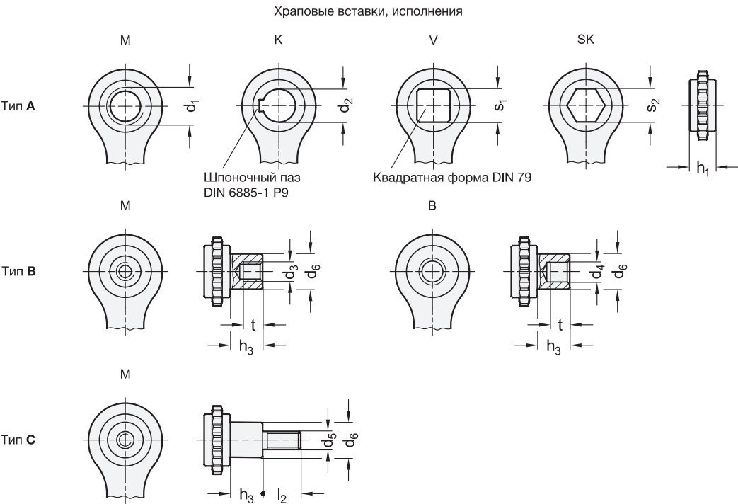
GN 318-Со сквозным отверстием / глухим отверстием STAINLESS STEEL
